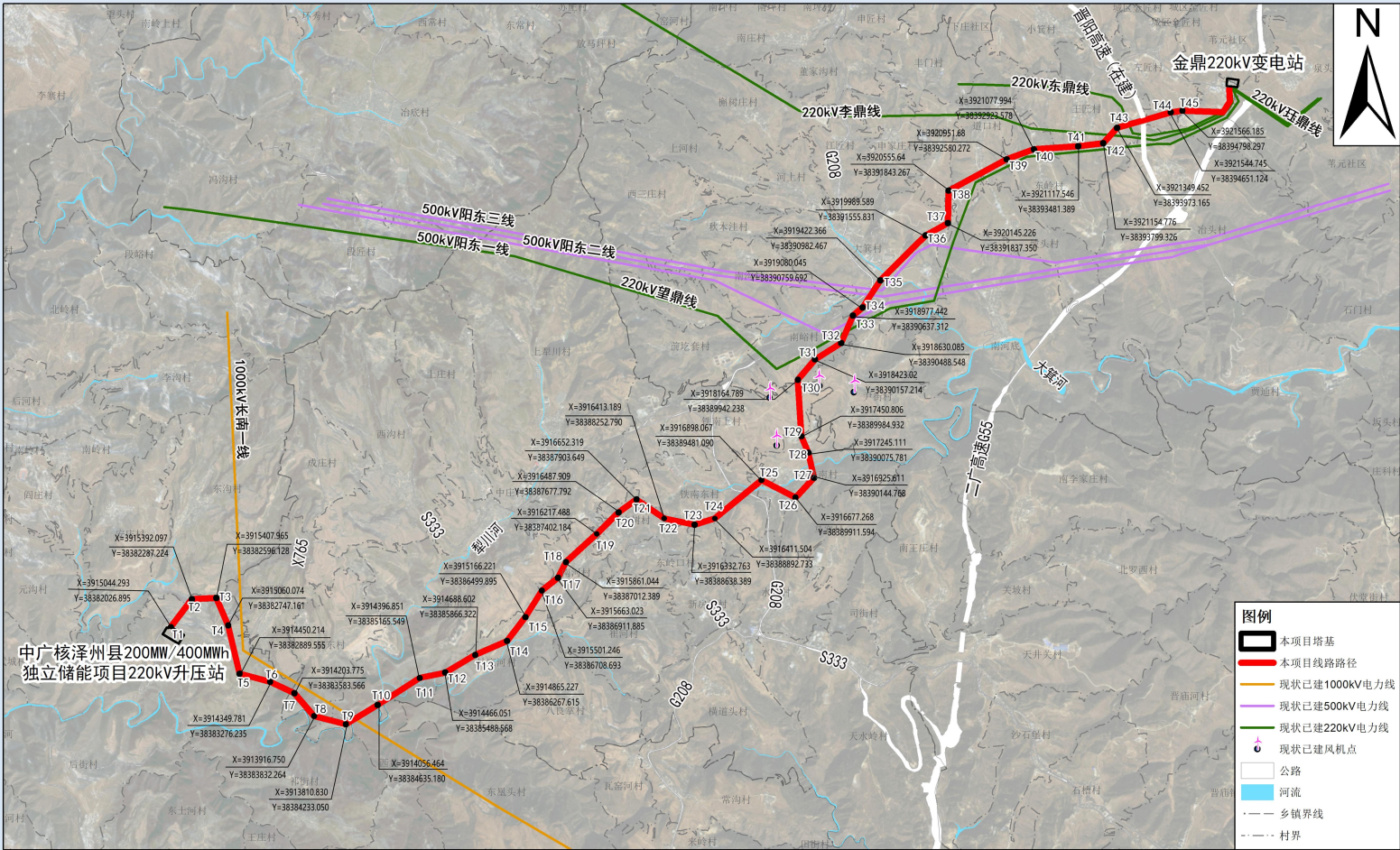
中广核泽州县200MW/400MWh独立储能项目220kV送出工程线路路径图
